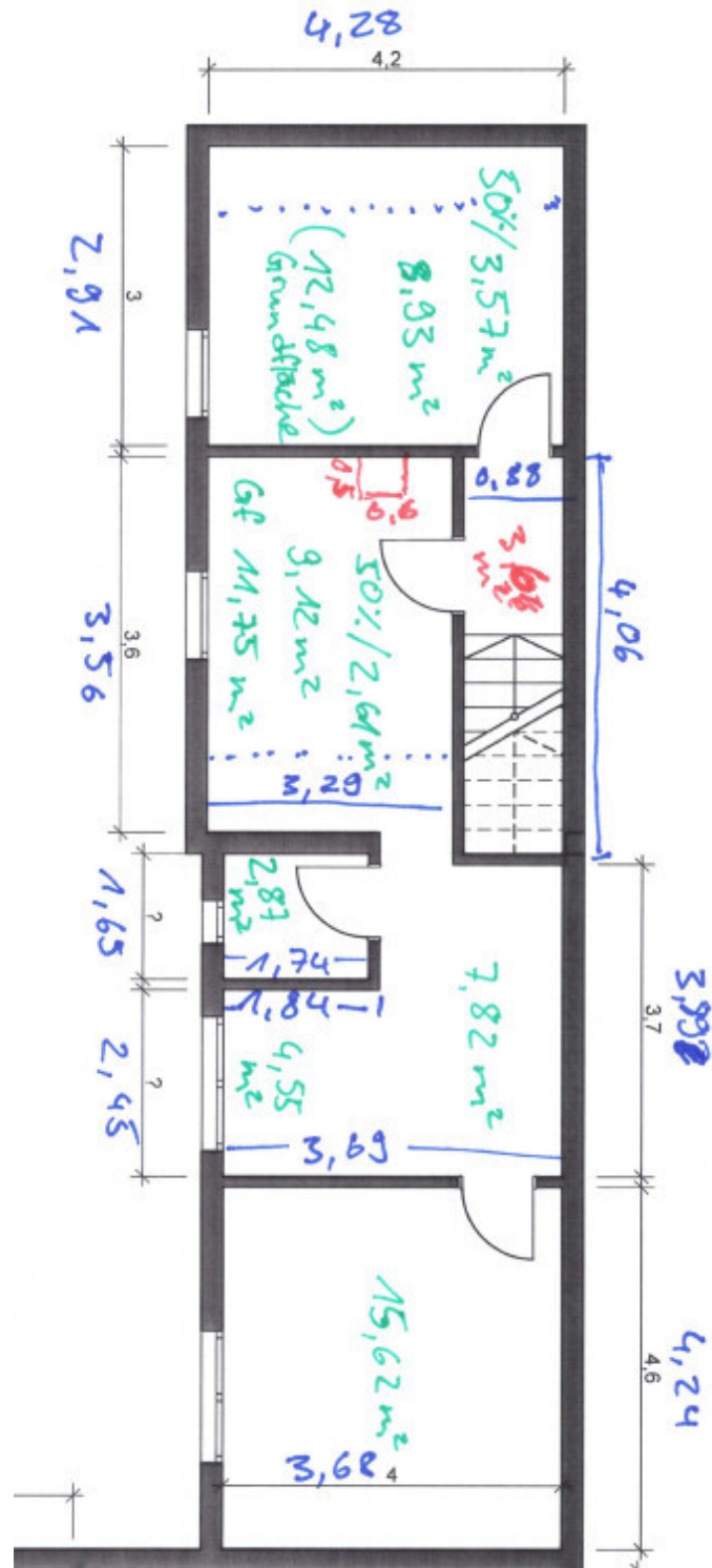
Skizze Grundriss OG Vorderhaus
